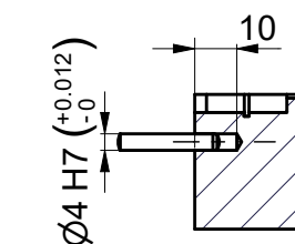
Section D-D
